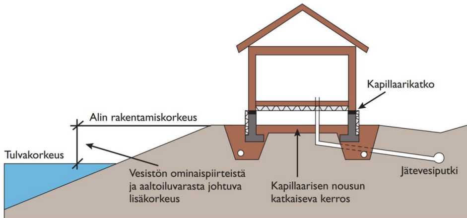
Kuva 2 Alin suositeltava rakentamiskorkeus tuulettuvalle alapohjalle. Lähde Ympäristöopas 2014.
