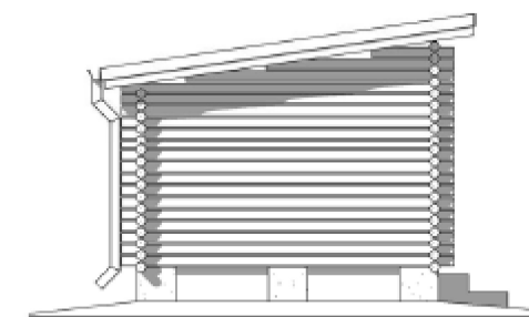
Julkisivu koilliseen
